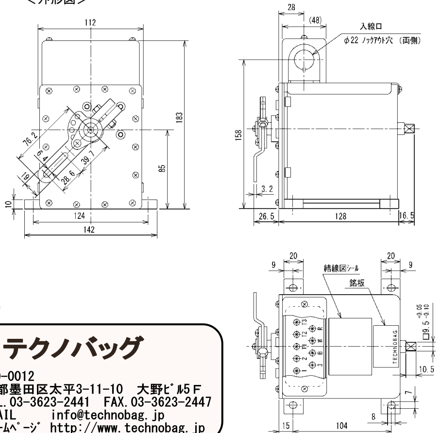
<外形図>
